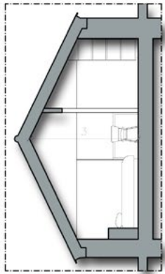
sezione B-B'
